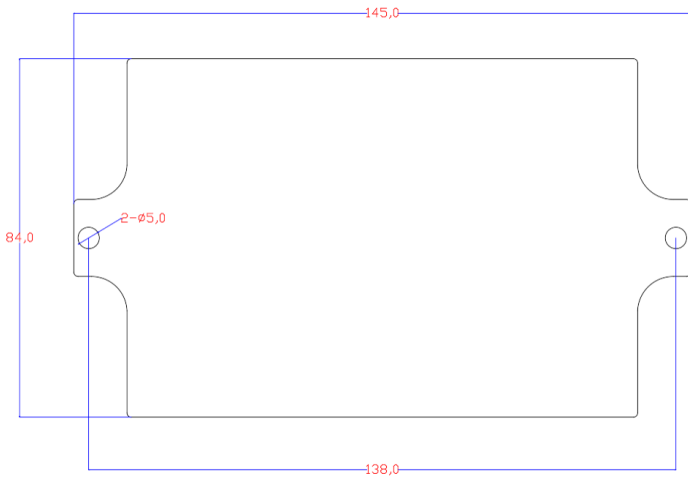
PM-CRADYBOX-AL-220X140X90 - 0186106
