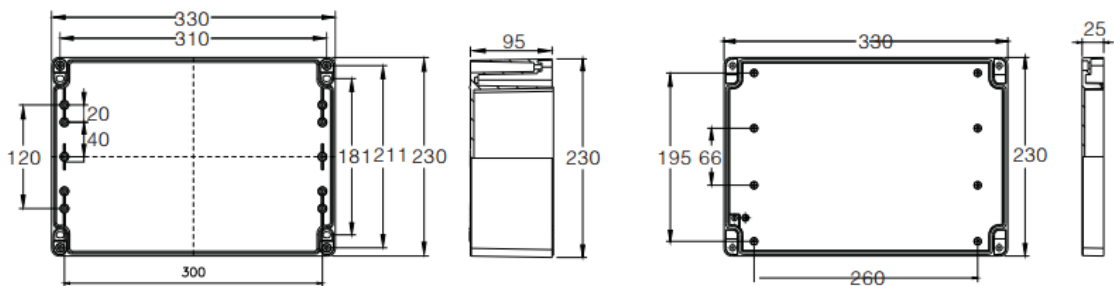
CRADYBOX-AL-330X230X120 - 0186008
