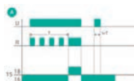
Retardo a la conexión
