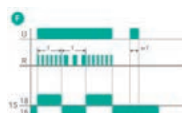
Ciclo simétrico, comienzo en on
