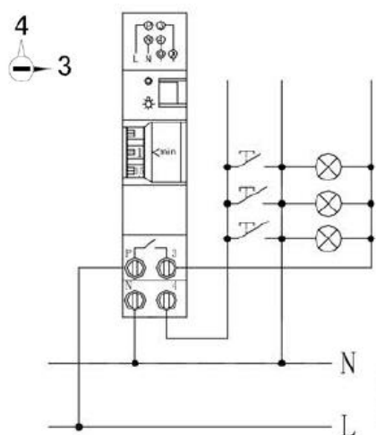
Conexión a 3 hilos
