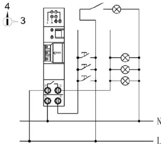
Conexión a 4 hilos
